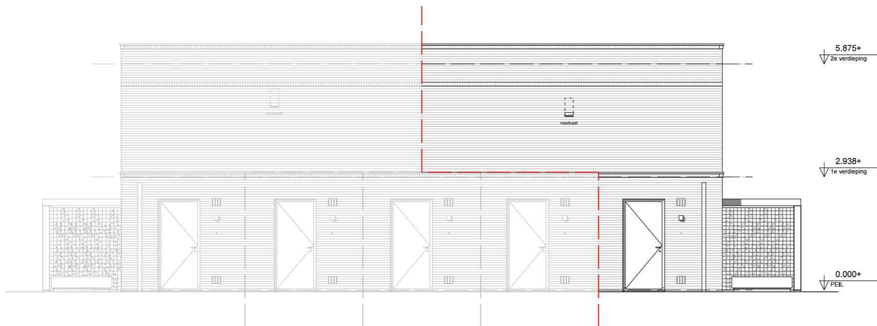
zijgevel
