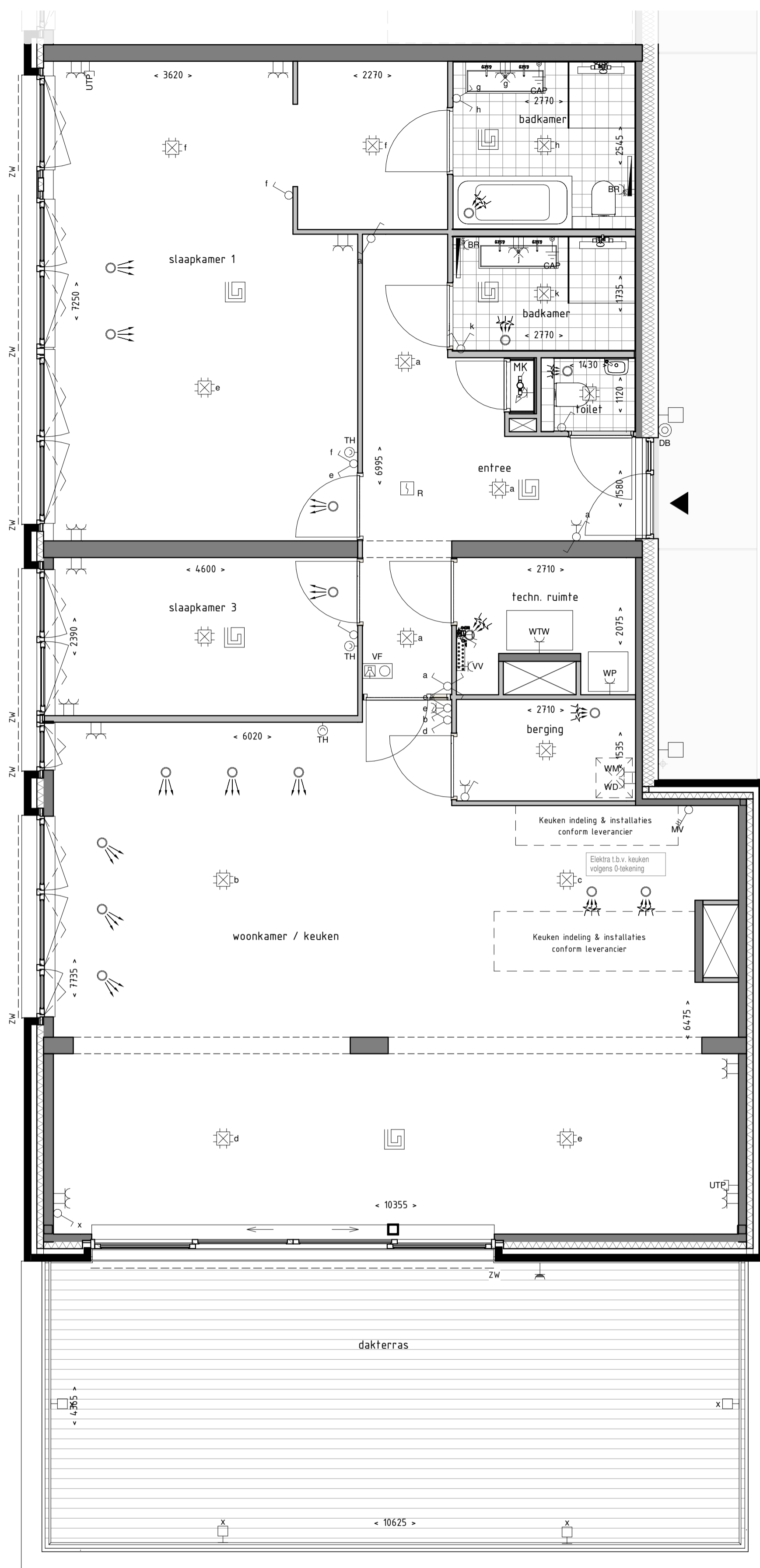
Optie 1 - 05.32.100 Slaapkamers samenvoegen
